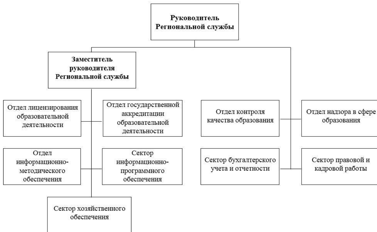
Рис. 2.1. Структура Ростобнадзора
